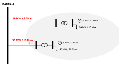
Figura 4 Sistema de potência a ser equivalentado - Geração
